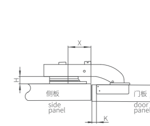
盖位计算值表 Calculation table of overlay
