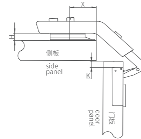
盖位计算值表 Calculation table of overlay
